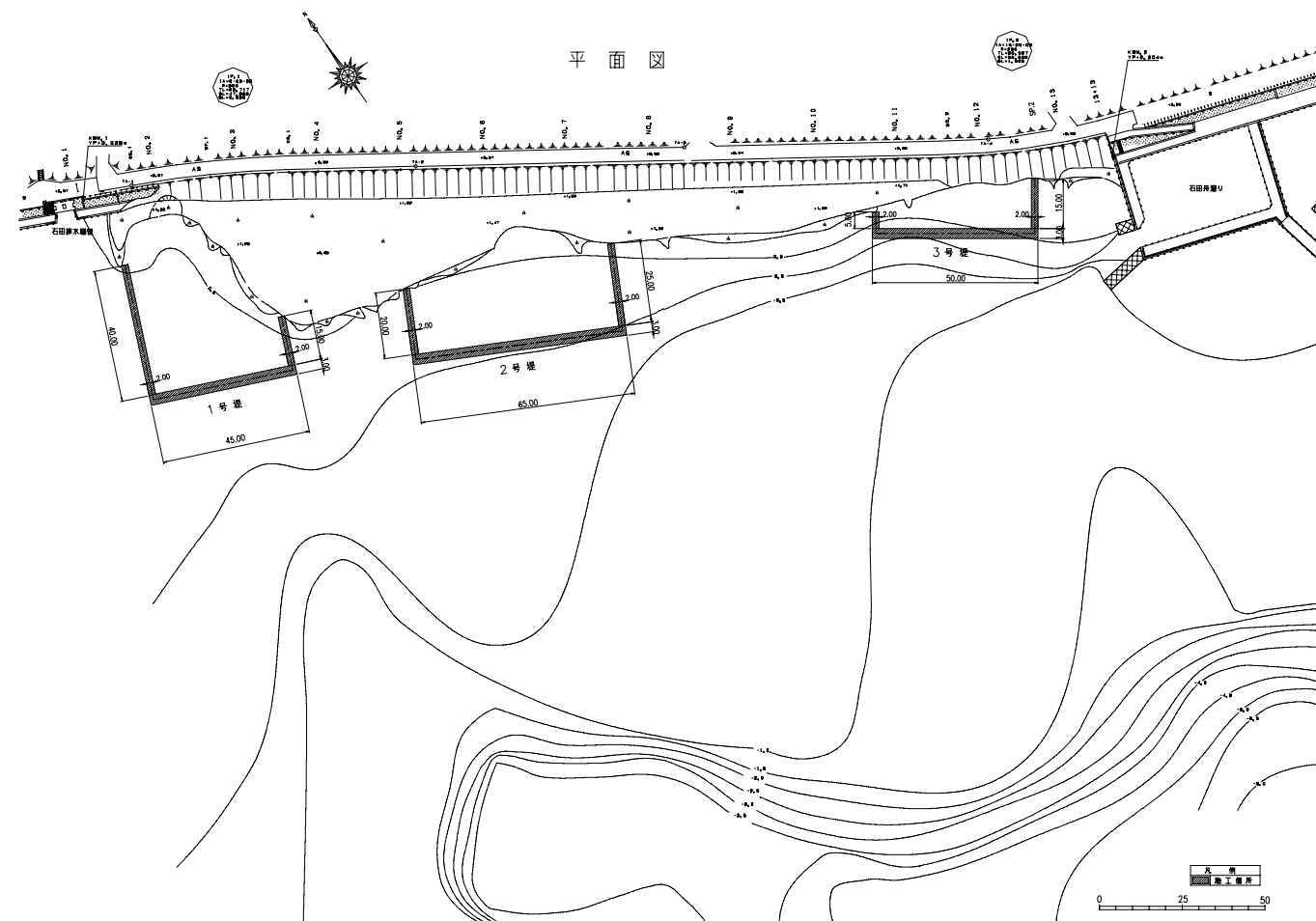
消波施設構造図(5) (2号堤)
