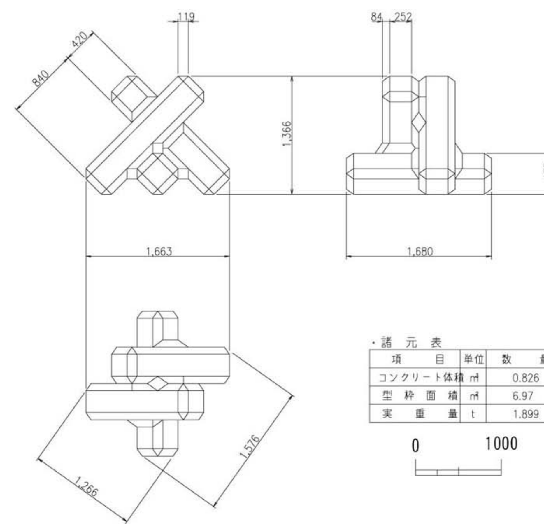
消波ブロック2t型構造図
