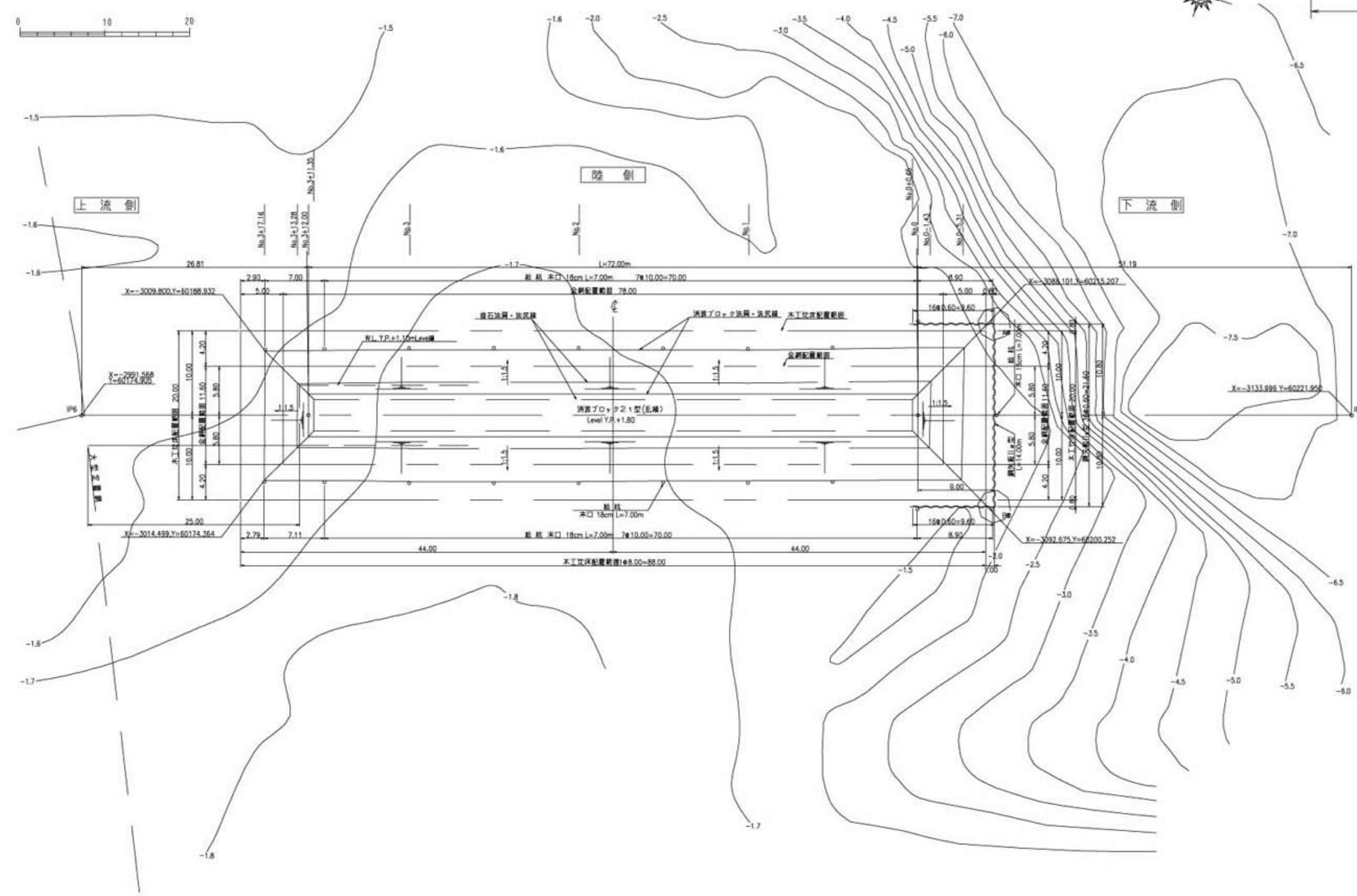
平面図(2)
