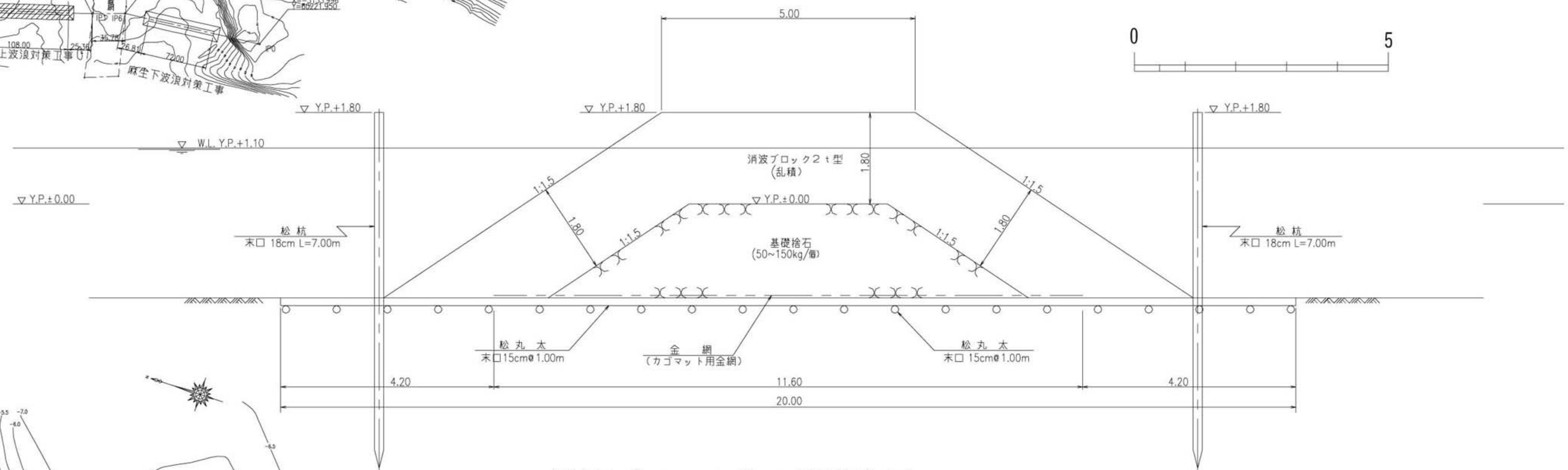
消波ブロック2t型構造図
