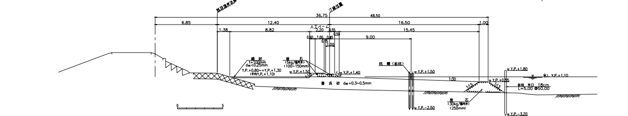
突堤工標準断面図 (突堤-1)
