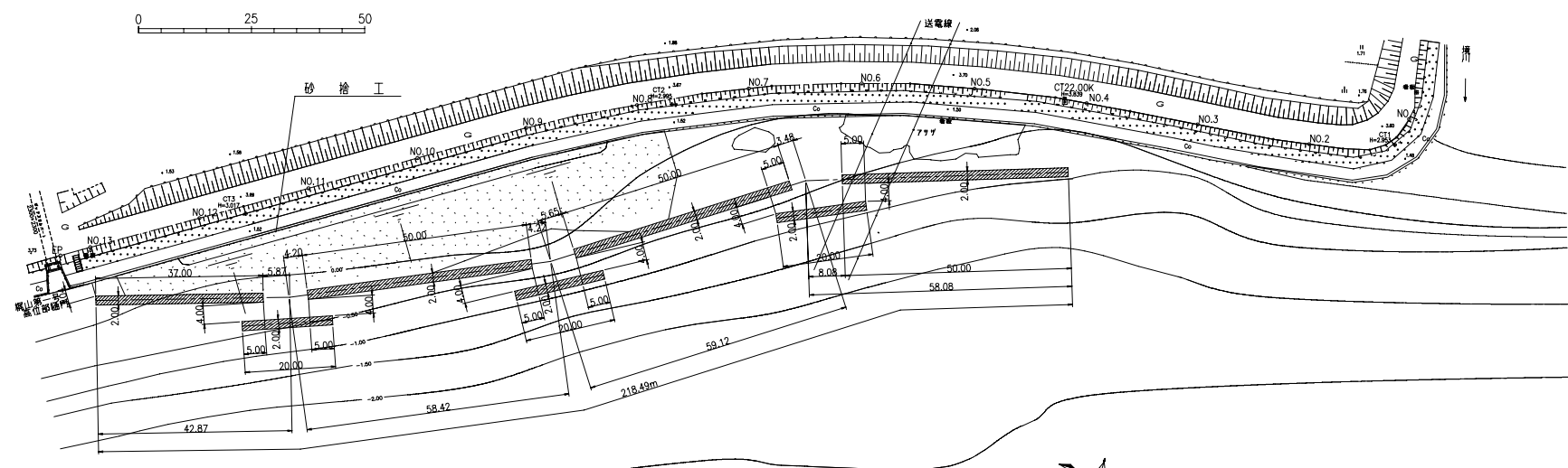
砂捨工平面図
